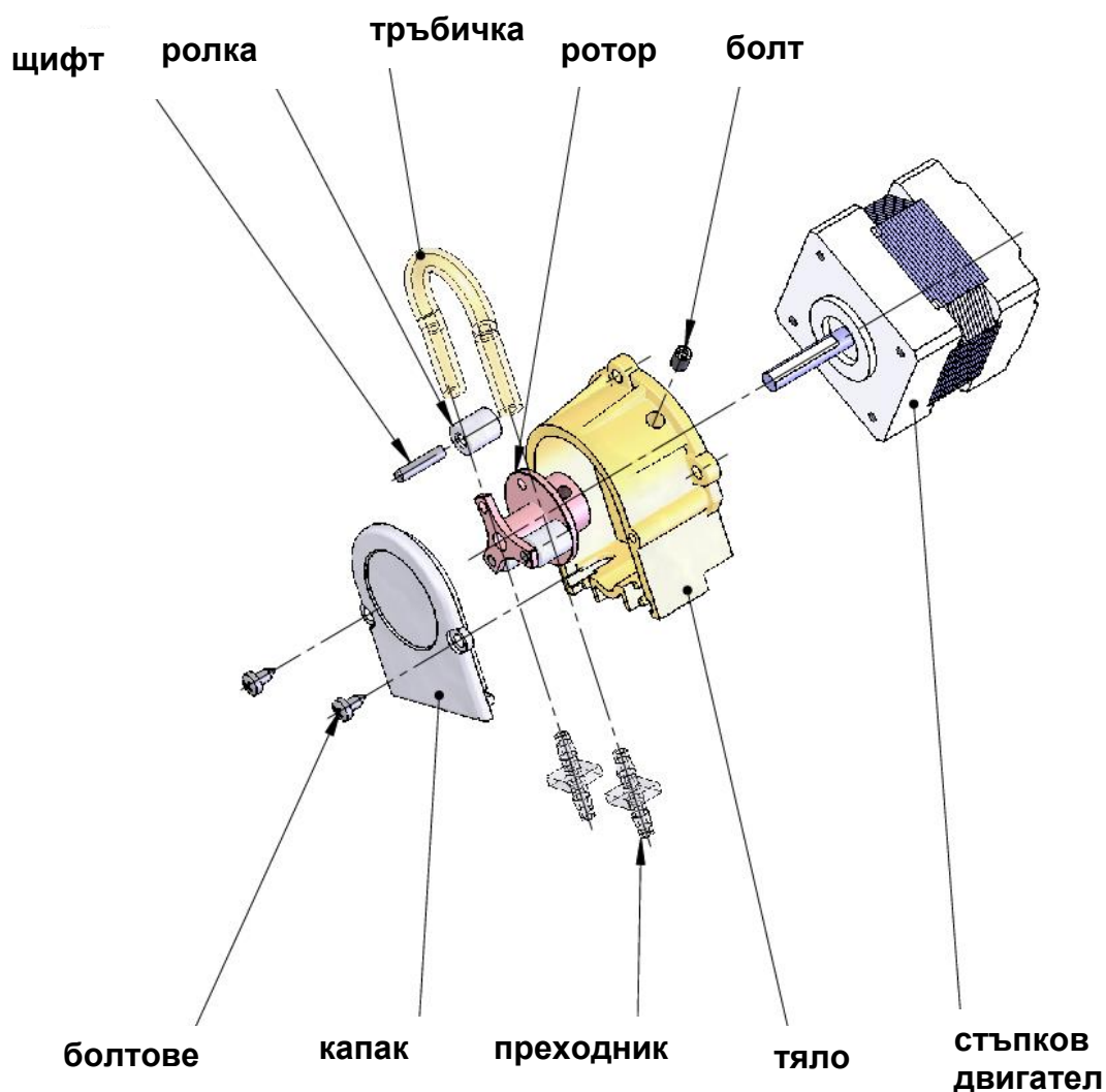
Фиг. 6 Перисталтична помпа
